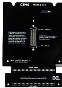
CB46 100-Pin Micro-D (Item 776)
